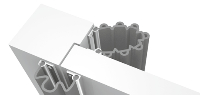
Coupe technique
