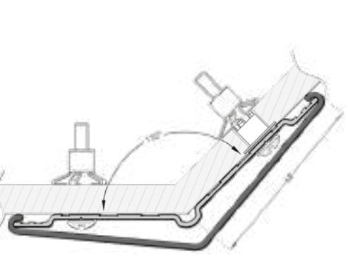
Coupe technique COMBO'CORNER 75 À 135°
